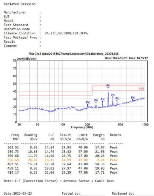
图 4-5 RE 测试水平方向
